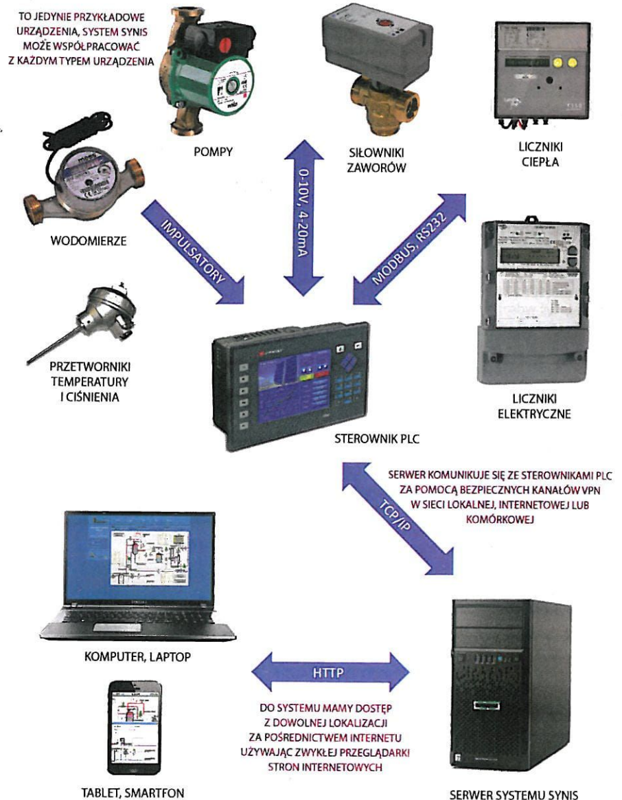
Rys. Uproszczony schemat budowy systemu SyNiS
